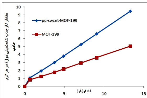
شکل ۷ نمودارهای هم‌دمای جذب گاز هیدروژن در دمای ۲۹۸ K و فشار ۱ تا ۱۵ bar بر روی نمونه‌های MOF-199 و Pd/SWCNTs@MOF-199
