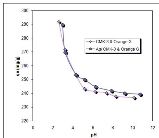
شکل ۸ اثر pH بر روی حذف رنگ اورانژ G به وسیله جاذب نانو ساختار CMK-3 و Ag/CMK-3 (غلظت ابتدای رنگ ۱۰۰۰ mg/l و مقدار مصرفی جاذب ۲۵ ml / ۵۰ mg، در دمای ۲۵ °C)
