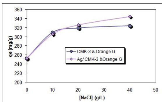
شکل ۸ اثر غلظت نمک بر روی حذف رنگ اورانژ G به وسیله جاذب نانو ساختار CMK-3 و Ag/CMK-3 (غلظت ابتدای رنگ 1000 \text{ mg/l} و مقدار مصرفی جاذب 25 \text{ ml} 25 \text{ mg} ، در دمای 25^\circ\text{C} )
