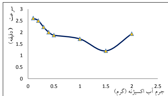
شکل ۶ تغییرات سرعت واکنش تشکیل ژل بر حسب مقدار آب اکسیژنه در محیط واکنش
