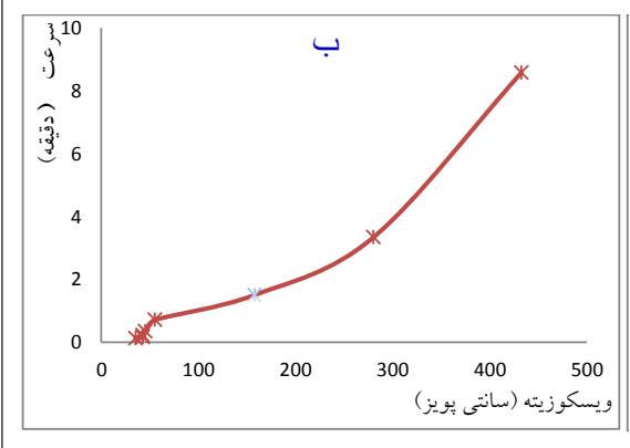
شکل ۵ تغییرات سرعت واکنش تشکیل بر حسب درصد گلیسرین (الف) و گرانیوی حلال (ب)
