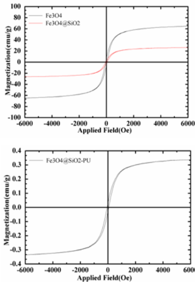
شکل ۷ منحنی ویژگی های مغناطیسی برای نانو ذرات Fe_3O_4 ، Fe_3O_4@SiO_2 و نانو کامپوزیت Fe_3O_4@SiO_2 -PU در دمای اتاق
