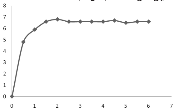
شکل ۹ بازده روغن هسته خرما در مقیاس نیم صنعتی (واریت زاهدی، S/L=3/1 ، حلال پترولیوم اتر و اندازه دانه‌های هسته ۱ mm)
