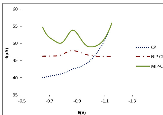
شکل ۴- مقایسه‌ی پاسخ SWV الکتروکدهای CP، NIP-CP، و MIP-CP پس از استخراج از محلول DZ M 5.0 \times 10^{-6} (pH=۳). (شرایط: Frequency = ۵۰ Hz t. step = ۰٫۳ s، \Delta E = 20 mv v. step = ۶ mv)
