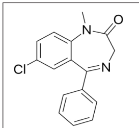
شکل ۱- ساختار شیمیایی مولکول دیاپام
