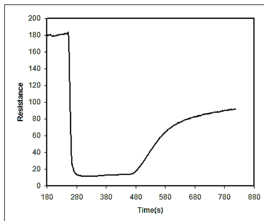
شکل ۷ رفتار پاسخ و بازیابی در نمونه روی اکسید همراه حاوی ۵ درصد لانتان نسبت به اتانول در دمای 350^{\circ}\text{C}
