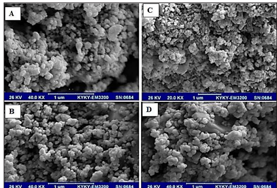
شکل ۳ تصویرهای SEM نانوکاتالیست‌های تهیه شده (Mg_{1-x}Zr_xNiO_3) (A) برابر با ۰، (B) برابر با ۰٫۱، (C) برابر با ۰٫۳ و (D) برابر با ۰٫۵
