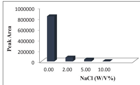
شکل ۶ تأثیر قدرت یونی بر کارایی استخراج OFL. شرایط آزمایش: ۱۰ ml محلول نمونه حاوی 500 \mu\text{g l}^{-1} OFL و 0.01 \text{ g} زوج یون \text{NaHxSo} , 150 \mu\text{l} حلال کلروفرم، زمان امولسیون‌سازی: ۳۰ ثانیه و زمان سانتریفوژ: ۵ دقیقه.
