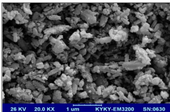
شکل ۳ تصویر SEM ترکیب نانوساختار (۱)
