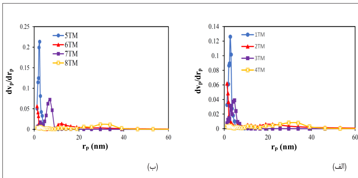
شکل ۴ نمودارهای توزیع اندازه حفره‌ها برای نمونه‌های تهیه شده با (الف) ۵ درصد مولی مینیزیم و (ب) ۱۵ درصد مولی مینیزیم
