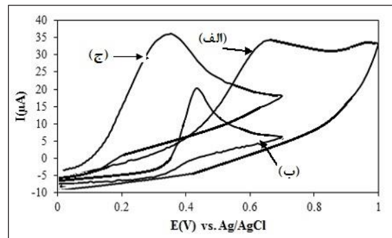
شکل ۱۰ ولتاموگرام اکسایش از: ال-سیستئین، (ب) اوریک اسید و (ج) آسکوربیک اسید، در محلول بافر فسفات ۰٫۱ M، pH=۷ با سرعت روبش ۱۰۰ mV/s
