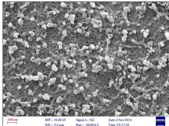
شکل ۲ تصویر میکروسکوپ الکترونی روبشی پلی‌ایندول/نانوذره‌های نقره
