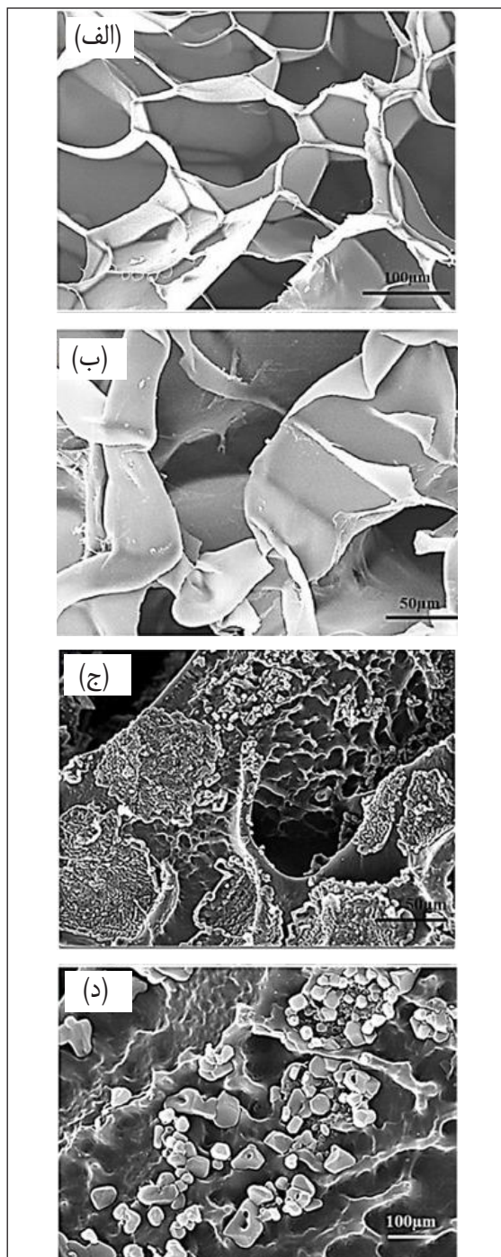
شکل ۴ تصاویر میکروسکوپ الکترونی روشی هیدروژل با بزرگنمایی (الف) ۹۰۰x، (ب) ۵۰۰x، حامل دارویی با بزرگنمایی (ج) ۹۰۰x و (د) ۳۰۰۰x
