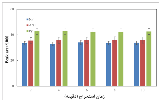
شکل ۳ تأثیر زمان بر بازده استخراج هیدروکربن‌های آروماتیک چندحلقه‌ای
